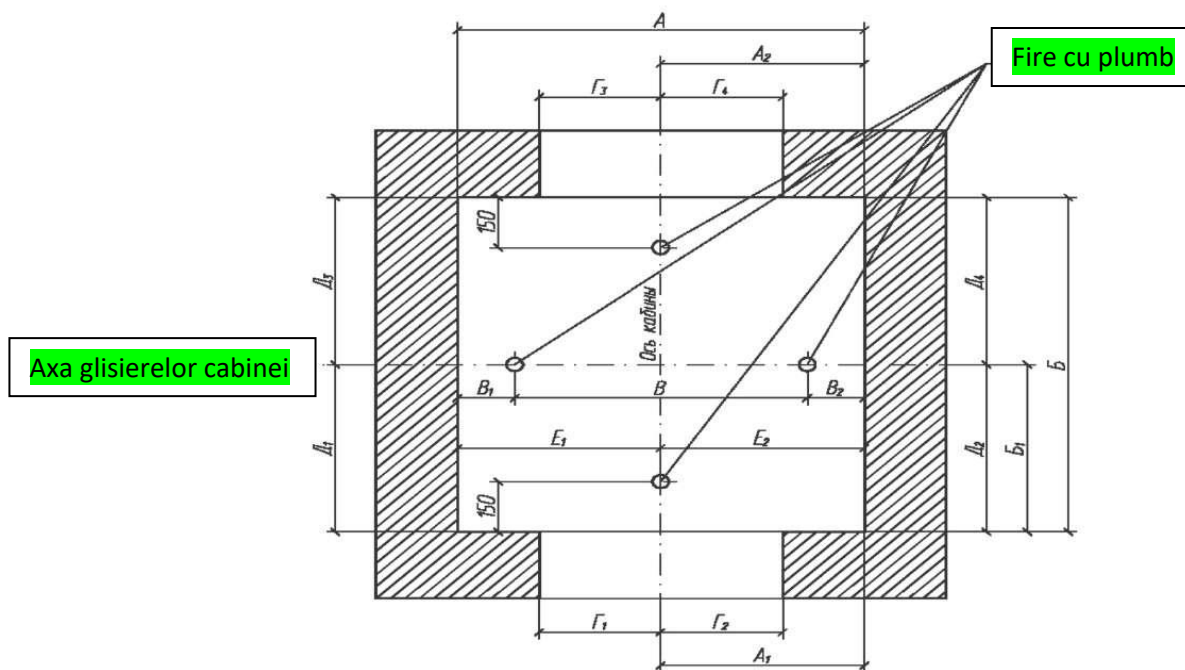
Figura A.1 - Schema executivă a părții de construcție a puțului ascensorului
