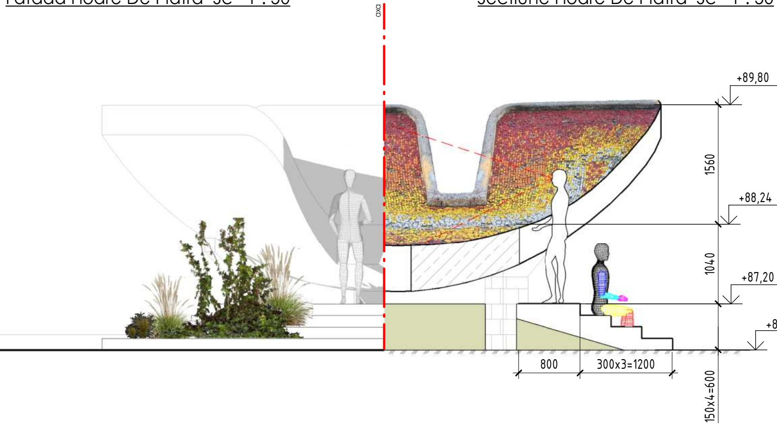
Fatada Floare De Piatră Sc 1 : 50
