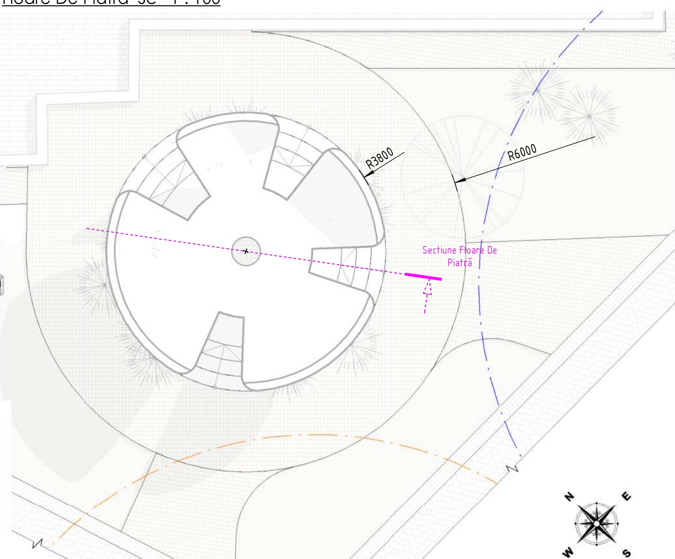
Floare De Piatră Sc 1 : 100
