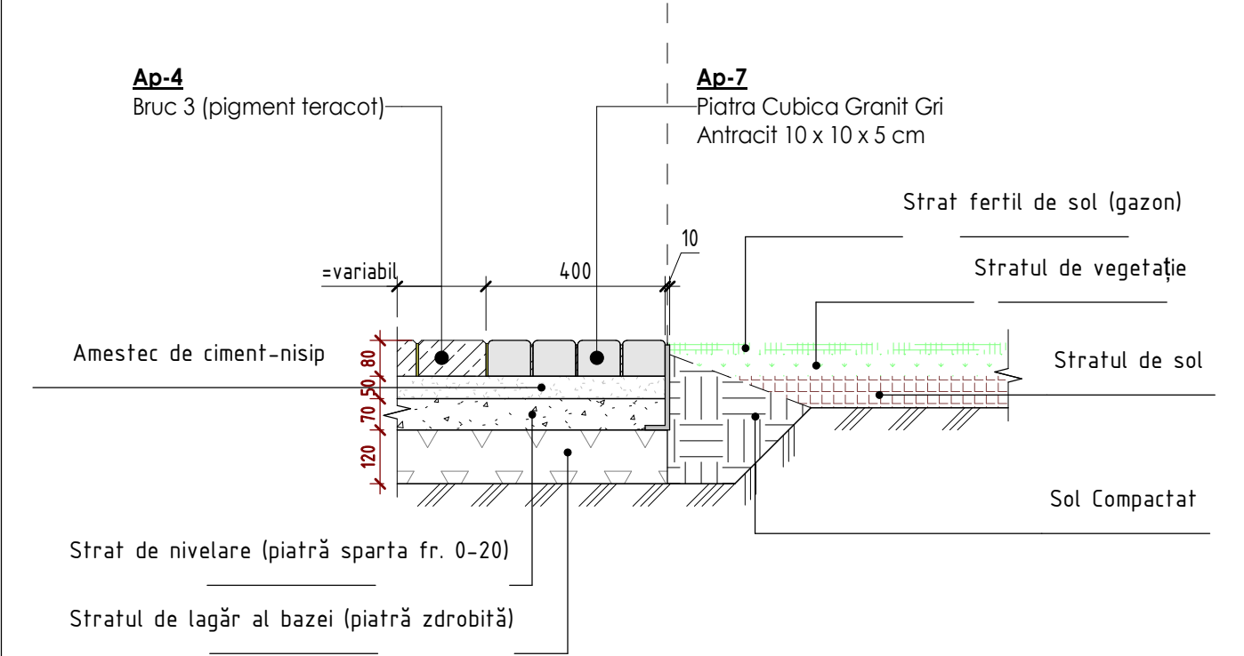
Nod acces pietonal (Bruc 3) Sc 1 : 15
